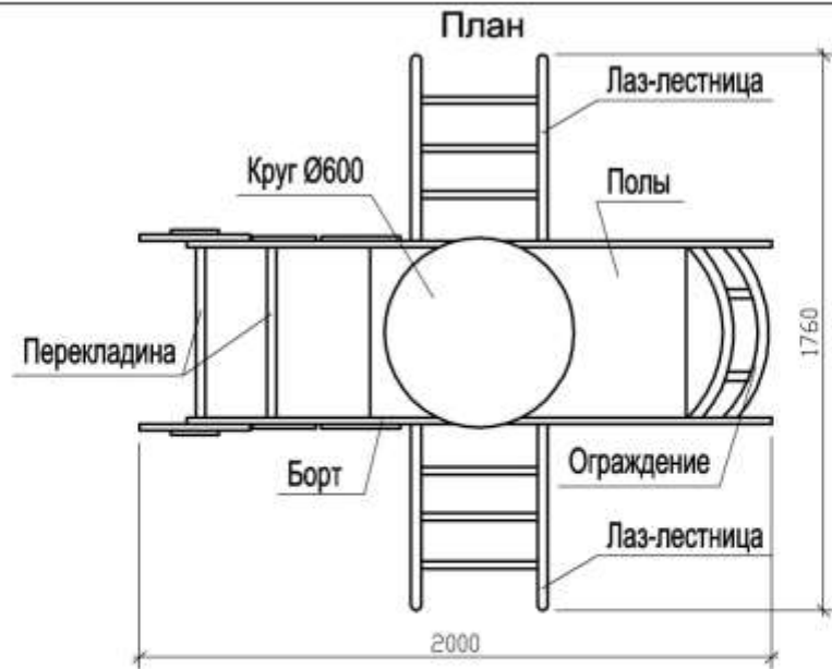
Схема расположения опор
